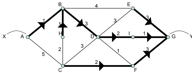
Arbre collecteur ayant G pour destination.
