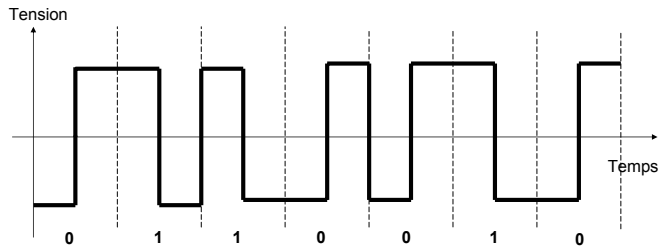
Code biphase (ou Manchester)
